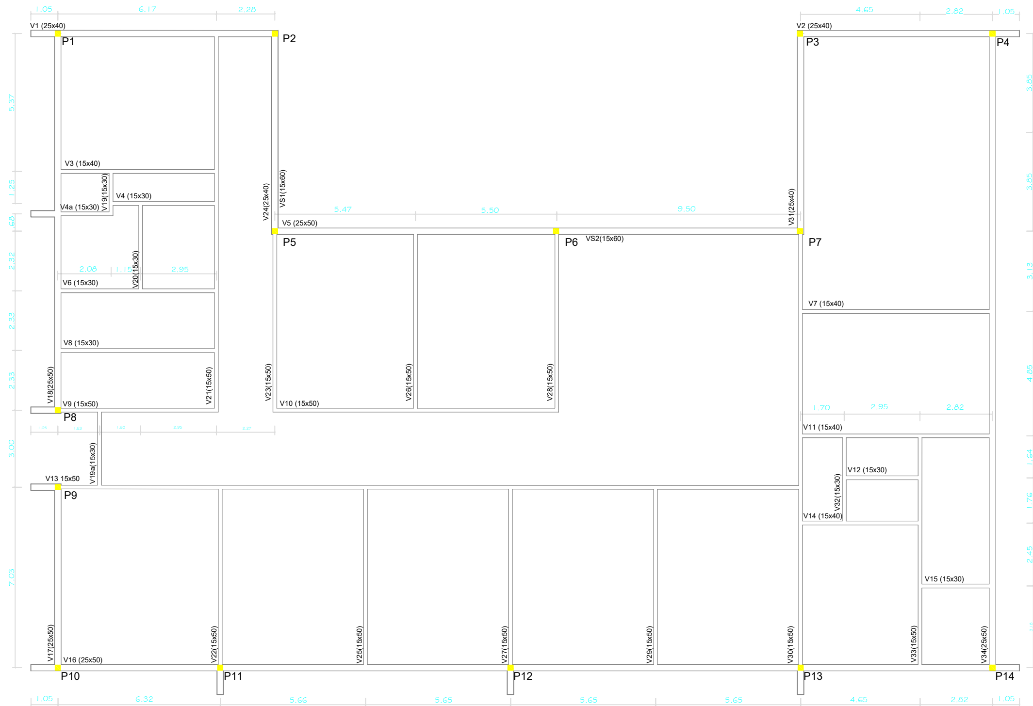
Locação de Vigas Baldrame, Pilares e Vigas Superiores Escala: 1/70
